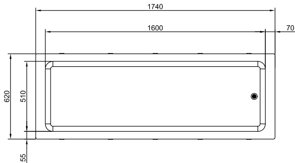
Päältä
